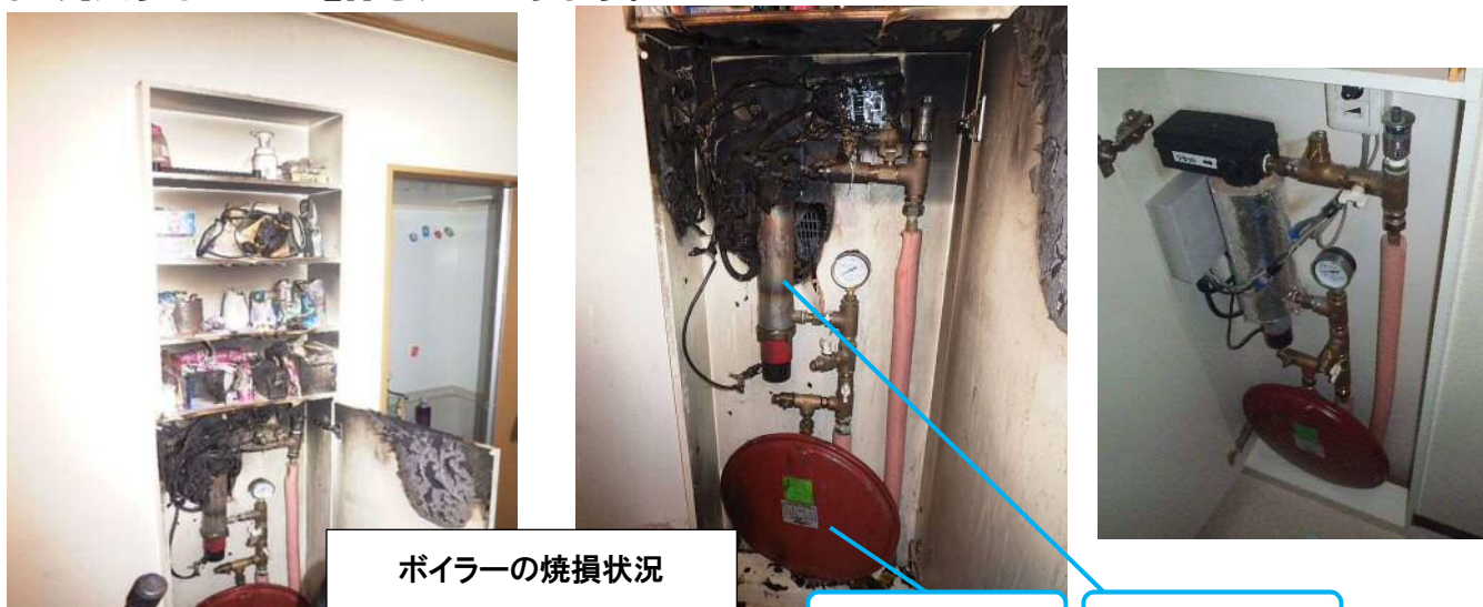
膨張タンク
